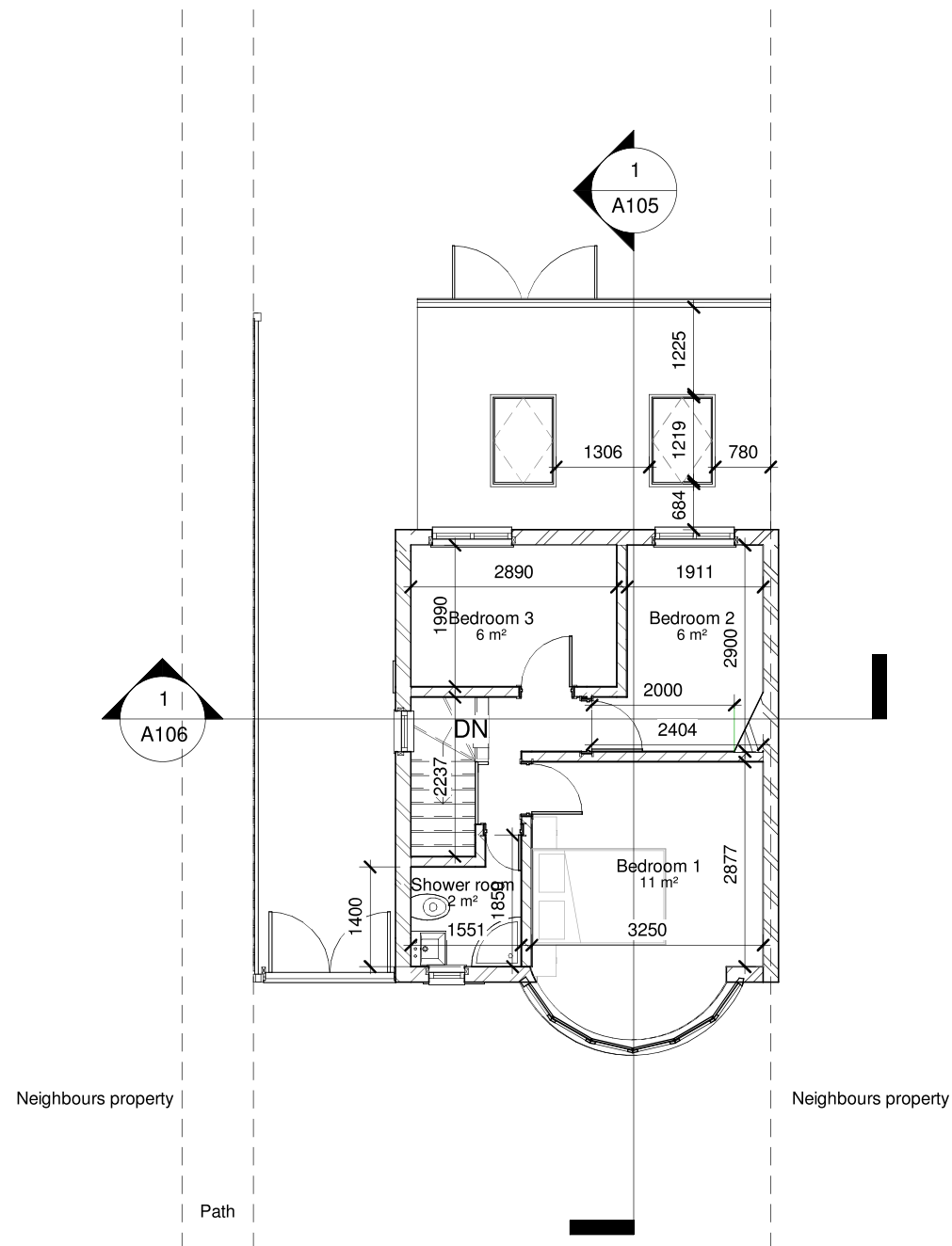
1 01- Existing 1 : 100
