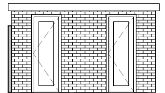
9 Garage Right 1 : 100
