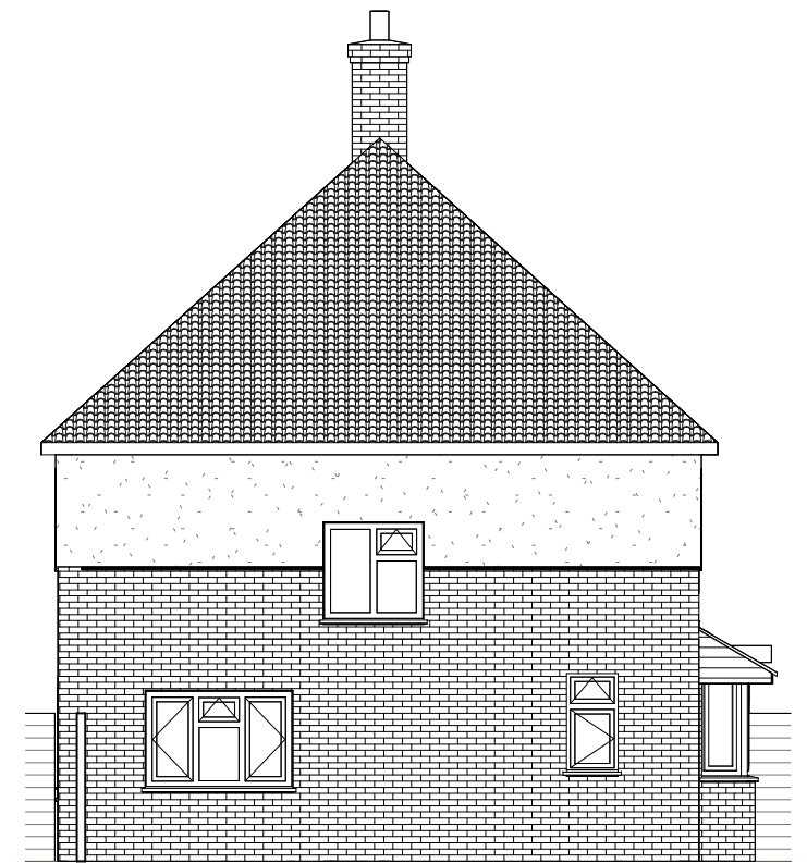
3 Left Elevation 1 : 100
