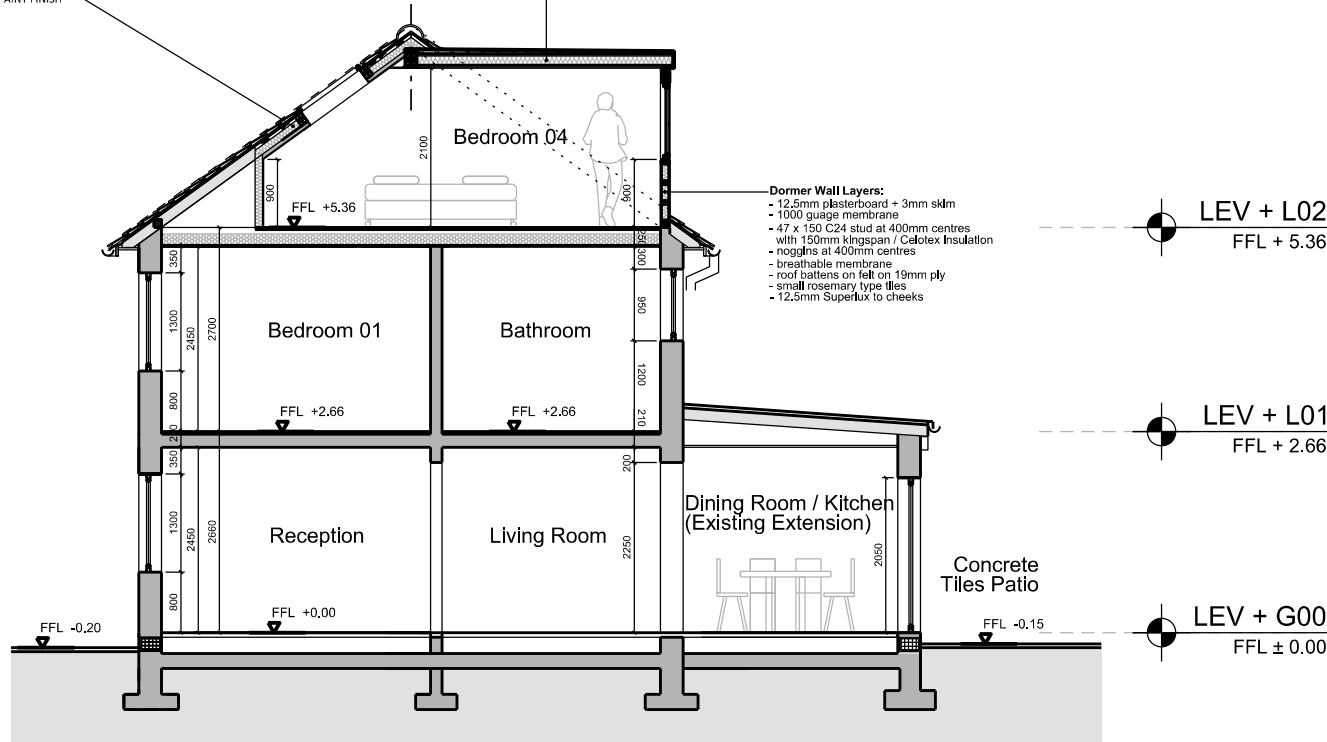
04 SECTION A-A 1:100
