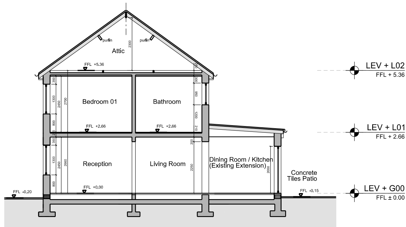
04 SECTION A-A 1:100
