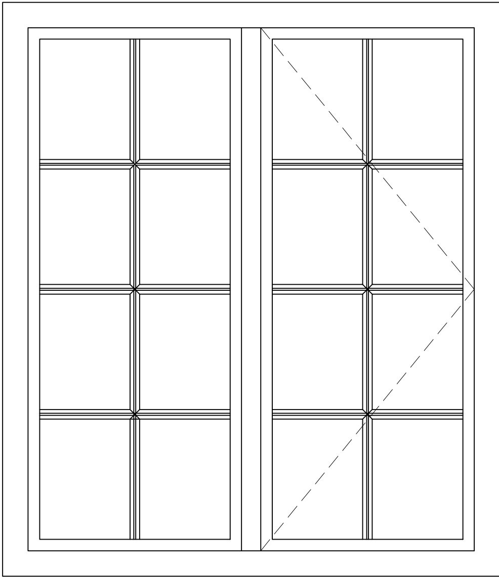
WINDOW ELEVATION SCALE: 1/10
