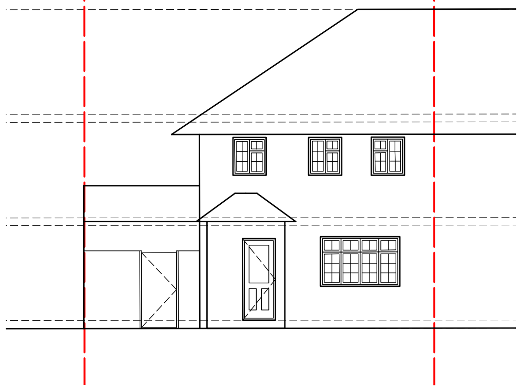
01 Front Elevation - Existing Scale: 1:100
