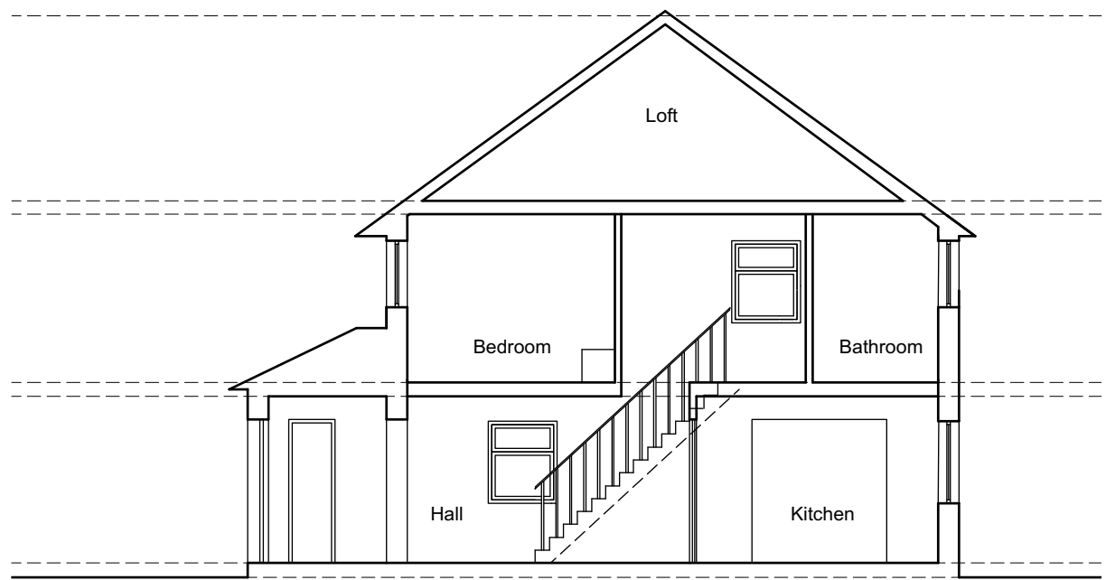
04 Section - Existing Scale: 1:100
