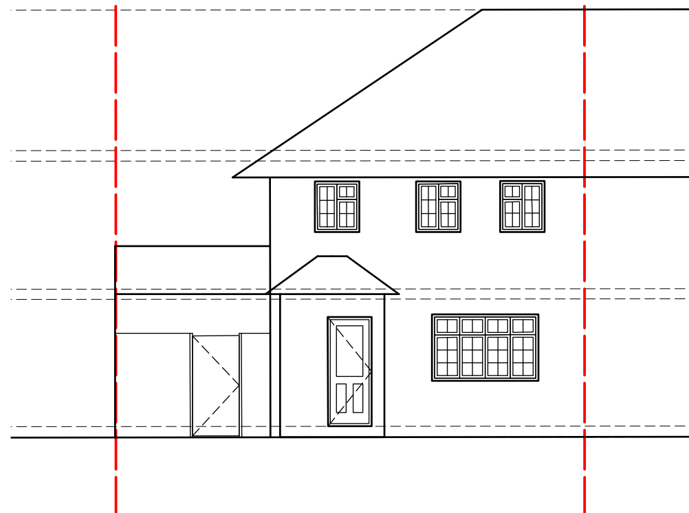
01 Front Elevation - Existing Scale: 1:100
