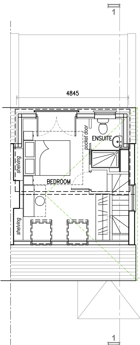
Loft Plan
