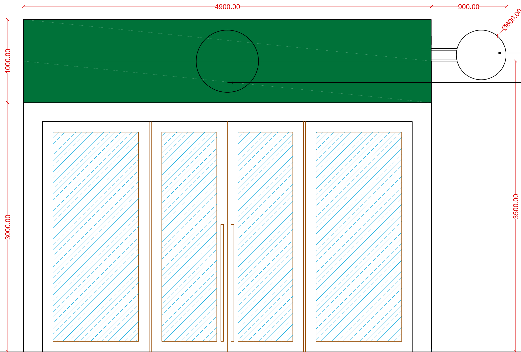
ELEVATION
