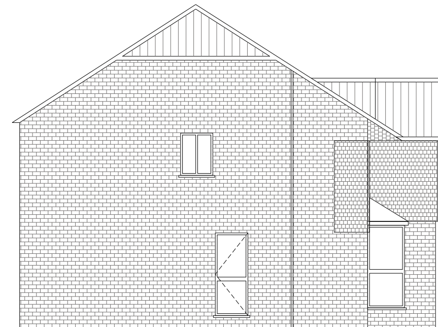
D. EXISTING SIDE ELEVATION
