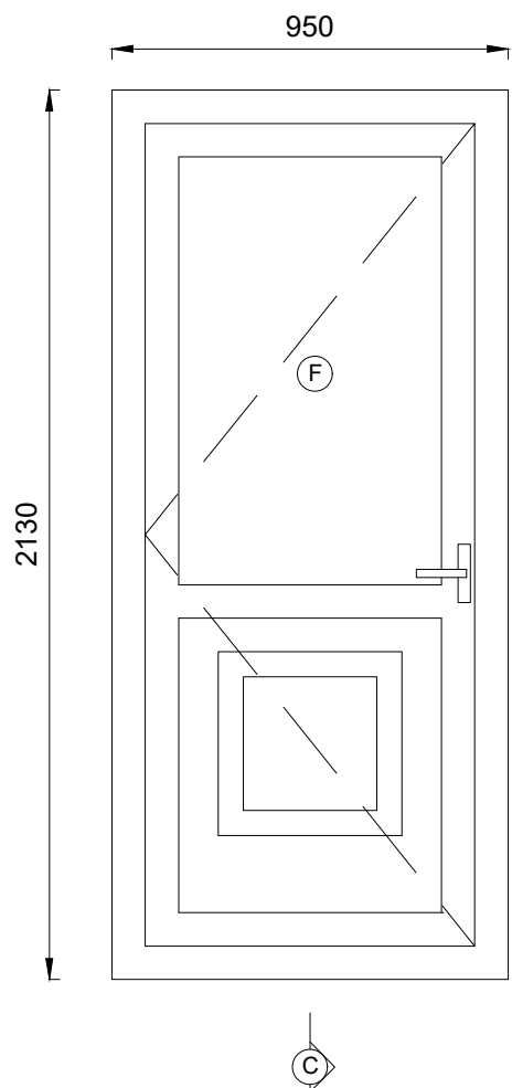
DOOR nos. 2,16,24,55 + 64 uPVC DOOR
