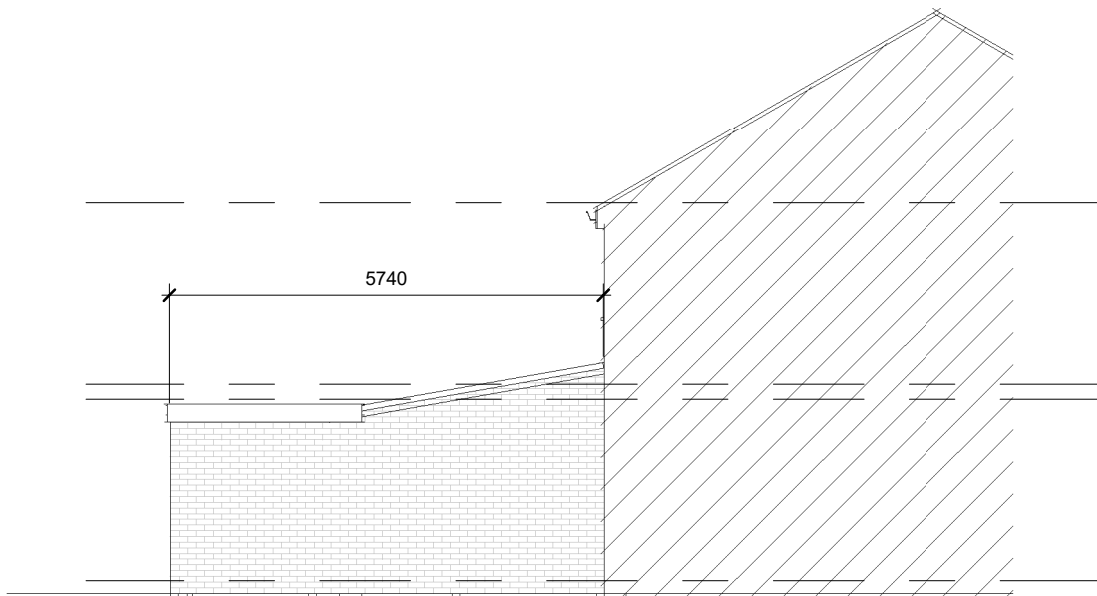
3 Left Elevation 1 : 100
