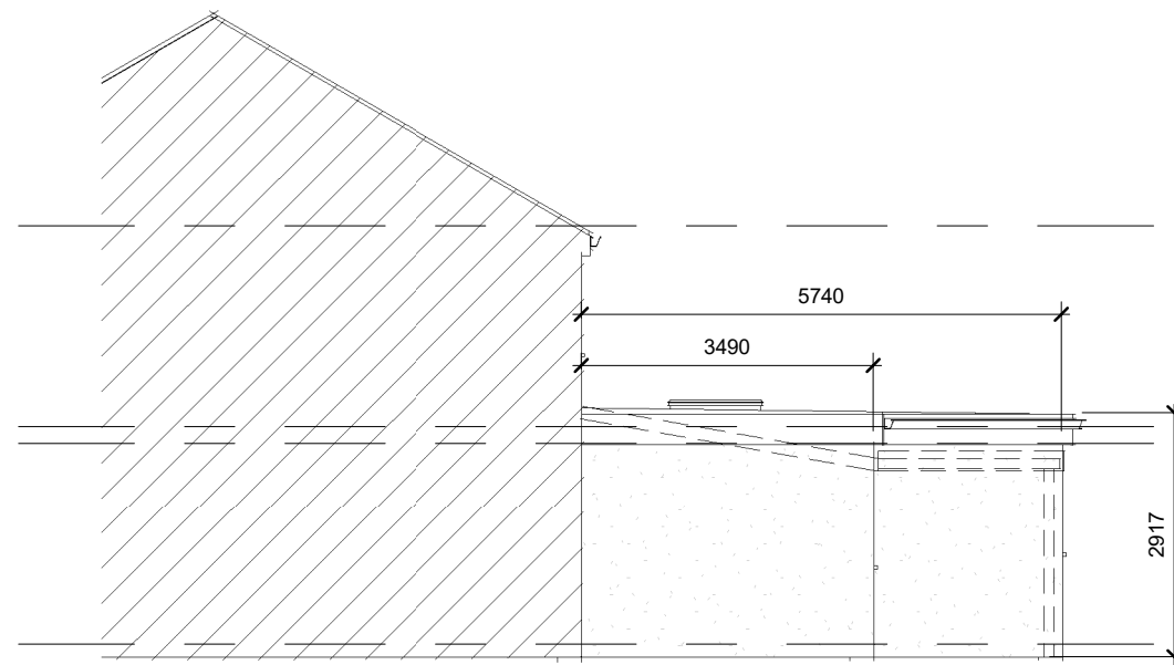
2 Right Elevation 1 : 100
