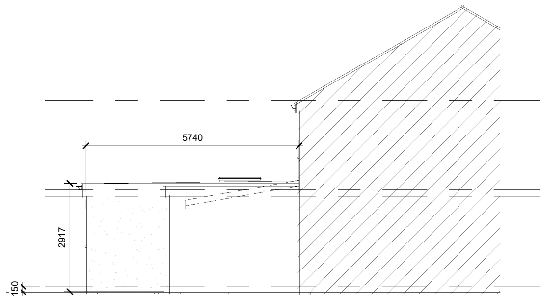
3 Left Elevation 1 : 100
