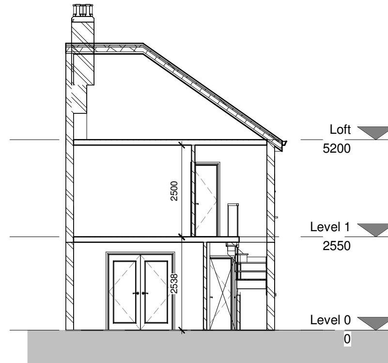
1 Existing - Section 1 1 : 100
