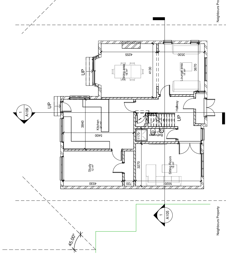
00 - Existing 1 : 100
