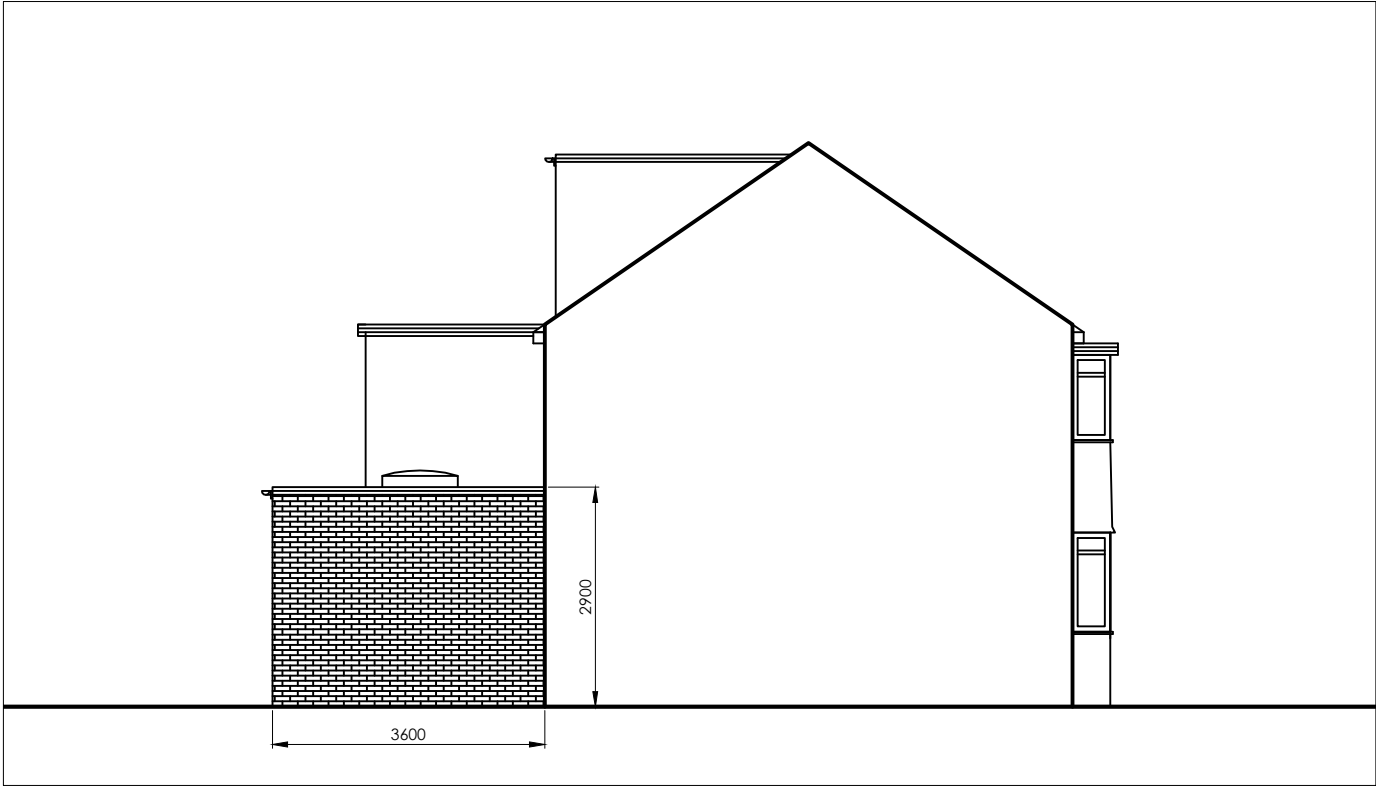
PROP SIDE ELEV
