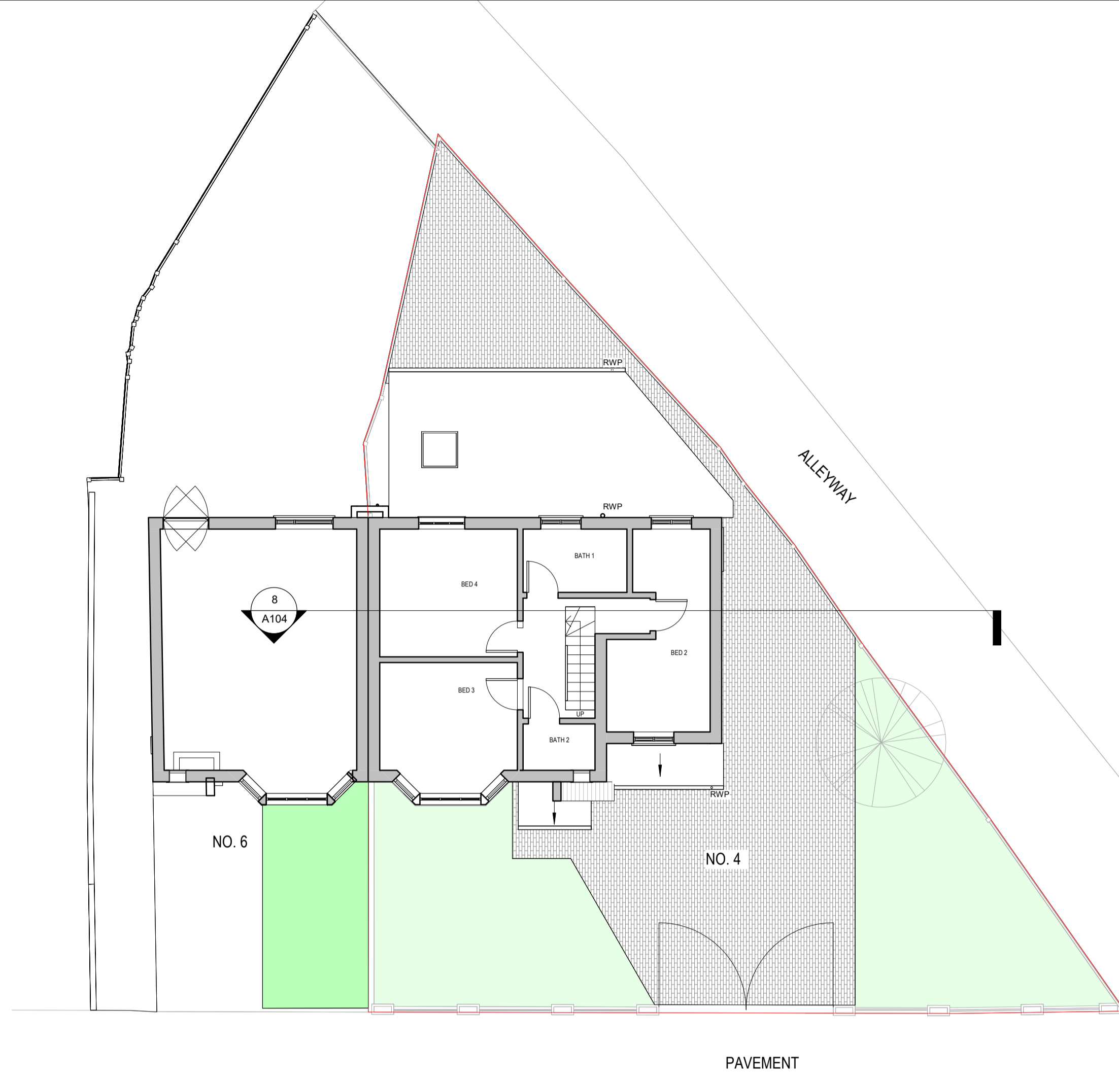
2 Existing FF Plan 1 : 100
