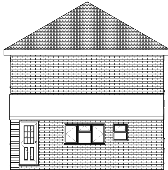
3 Left Existing 1 : 100
