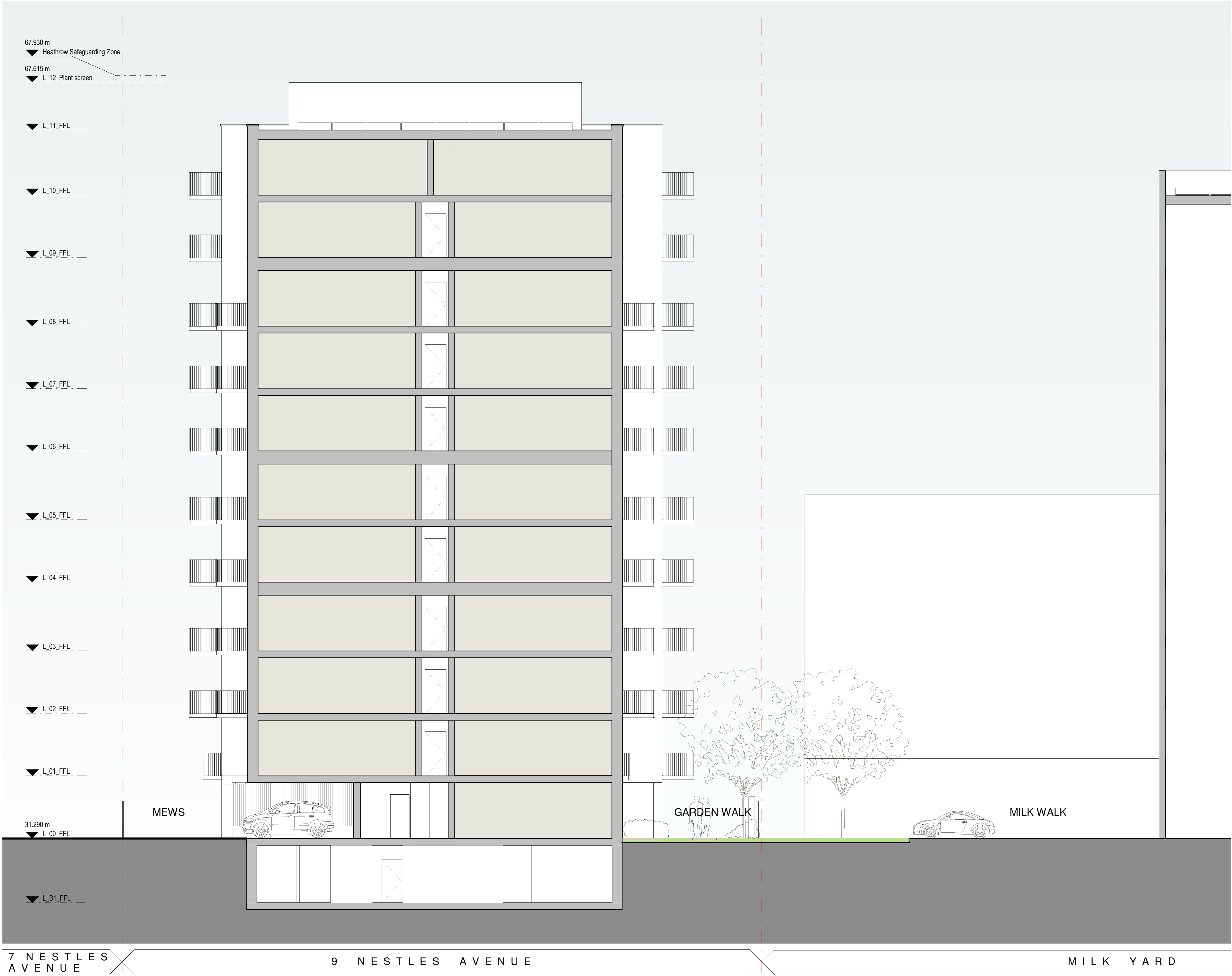
1 Section AA 1 : 100
