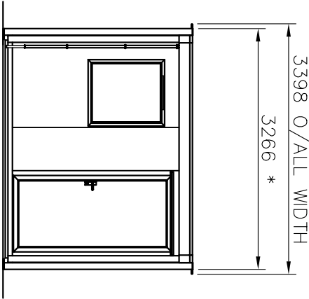
END ELEVATION
