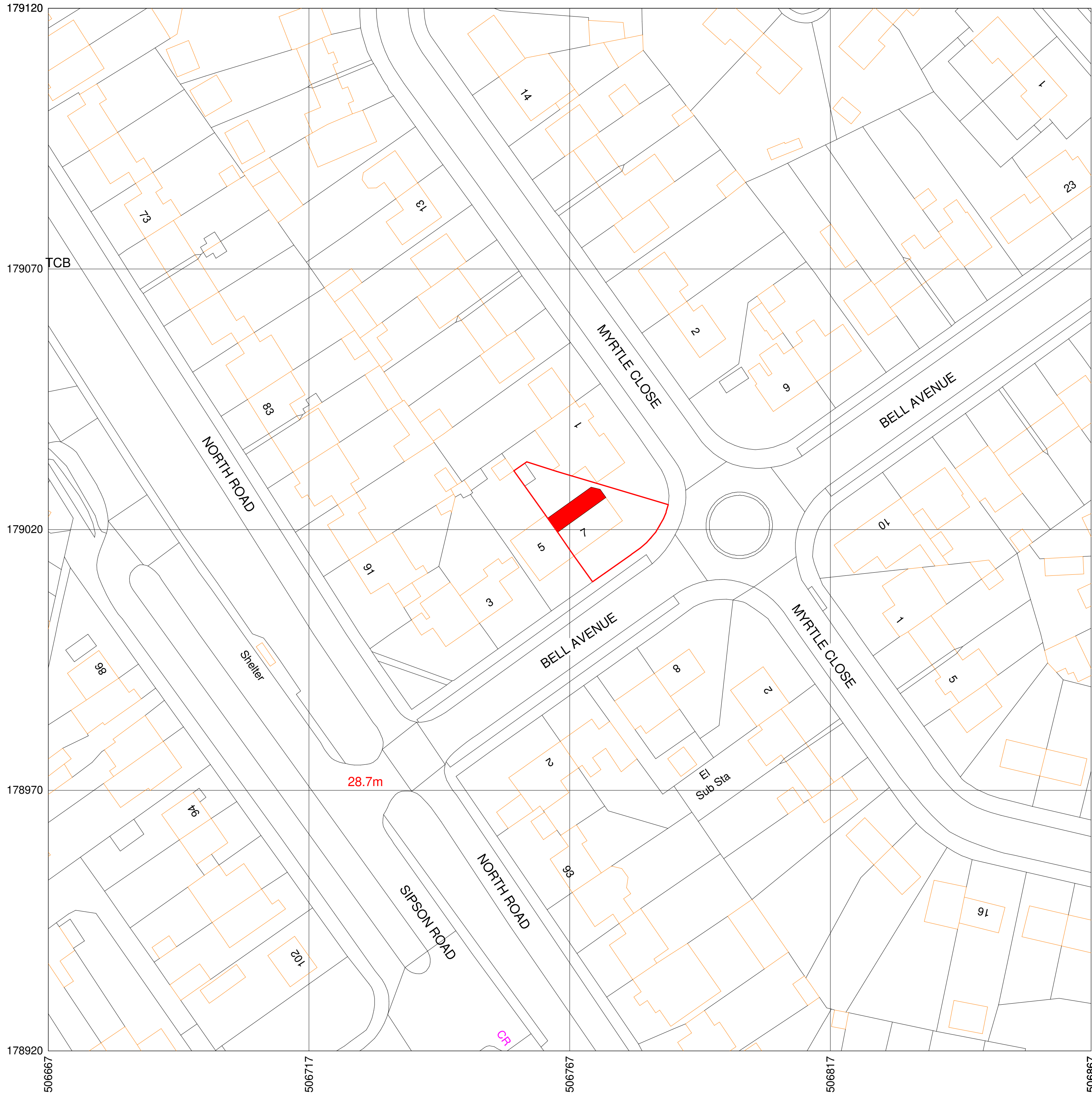
1 Block Plan 1 : 500
