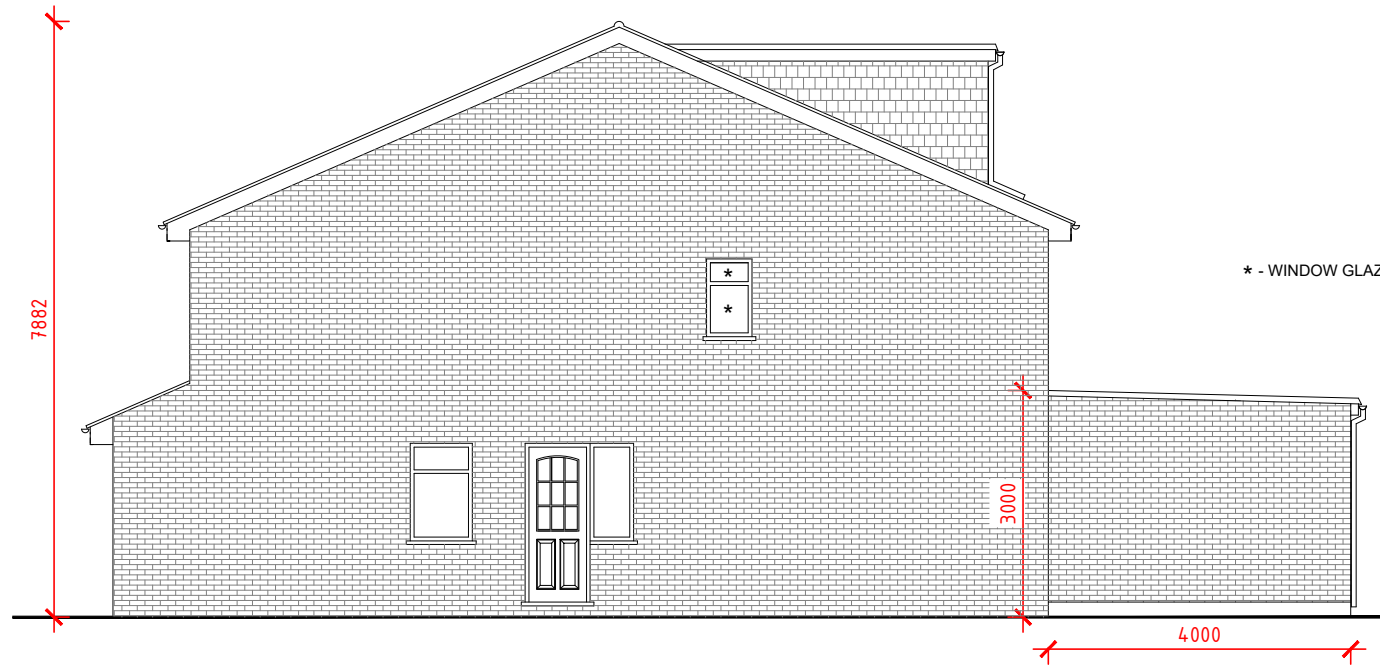
RIGHT ELEVATION
