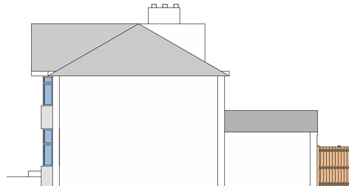
Elevation B
