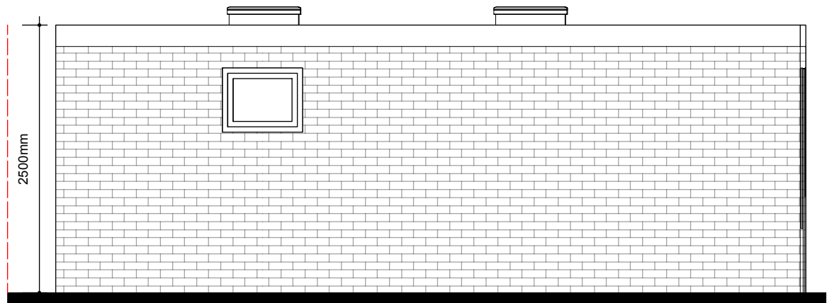
4 Side Elevation 1:50
