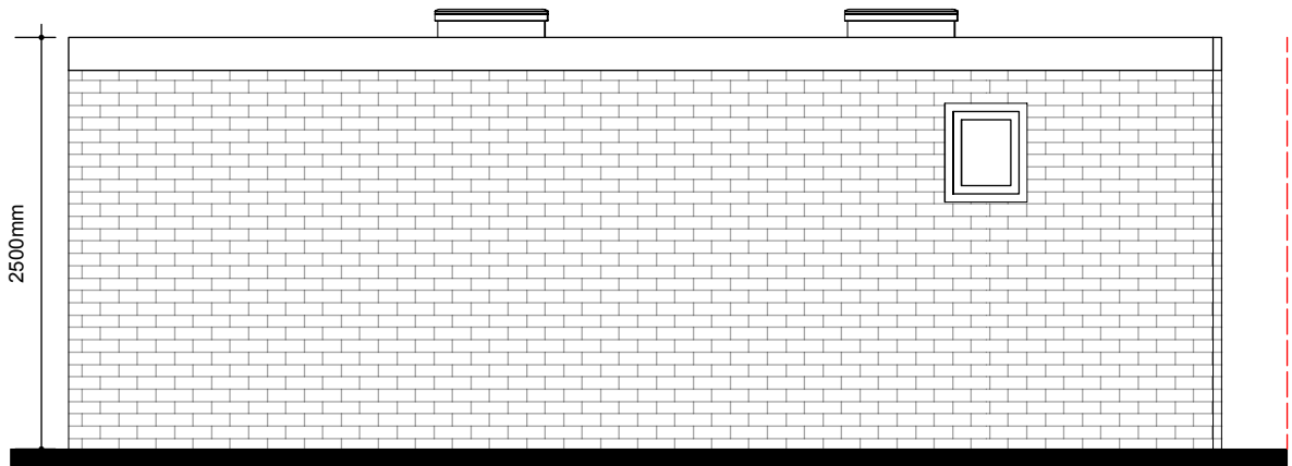
2 Side Elevation 1:50
