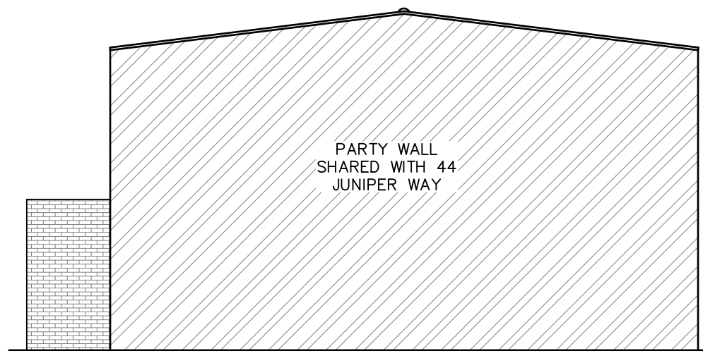
EXISTING FLANK ELEVATION
