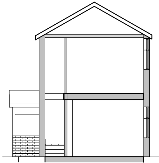
1 EXISTING SECTION 1 : 100
