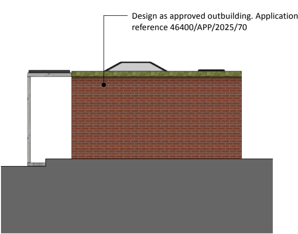
2 EAST Scale: 1:100
