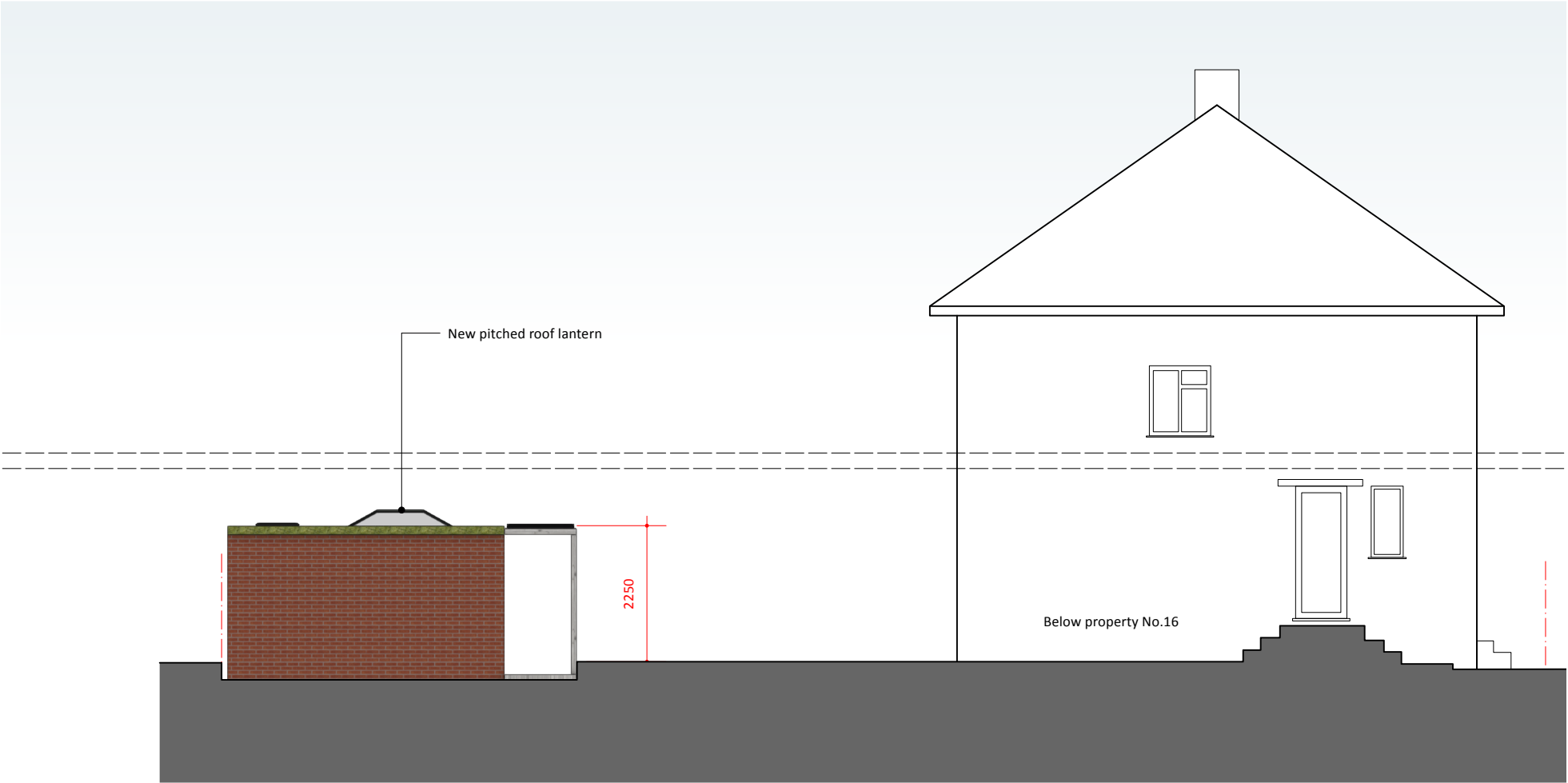
1 WEST Scale: 1:100
