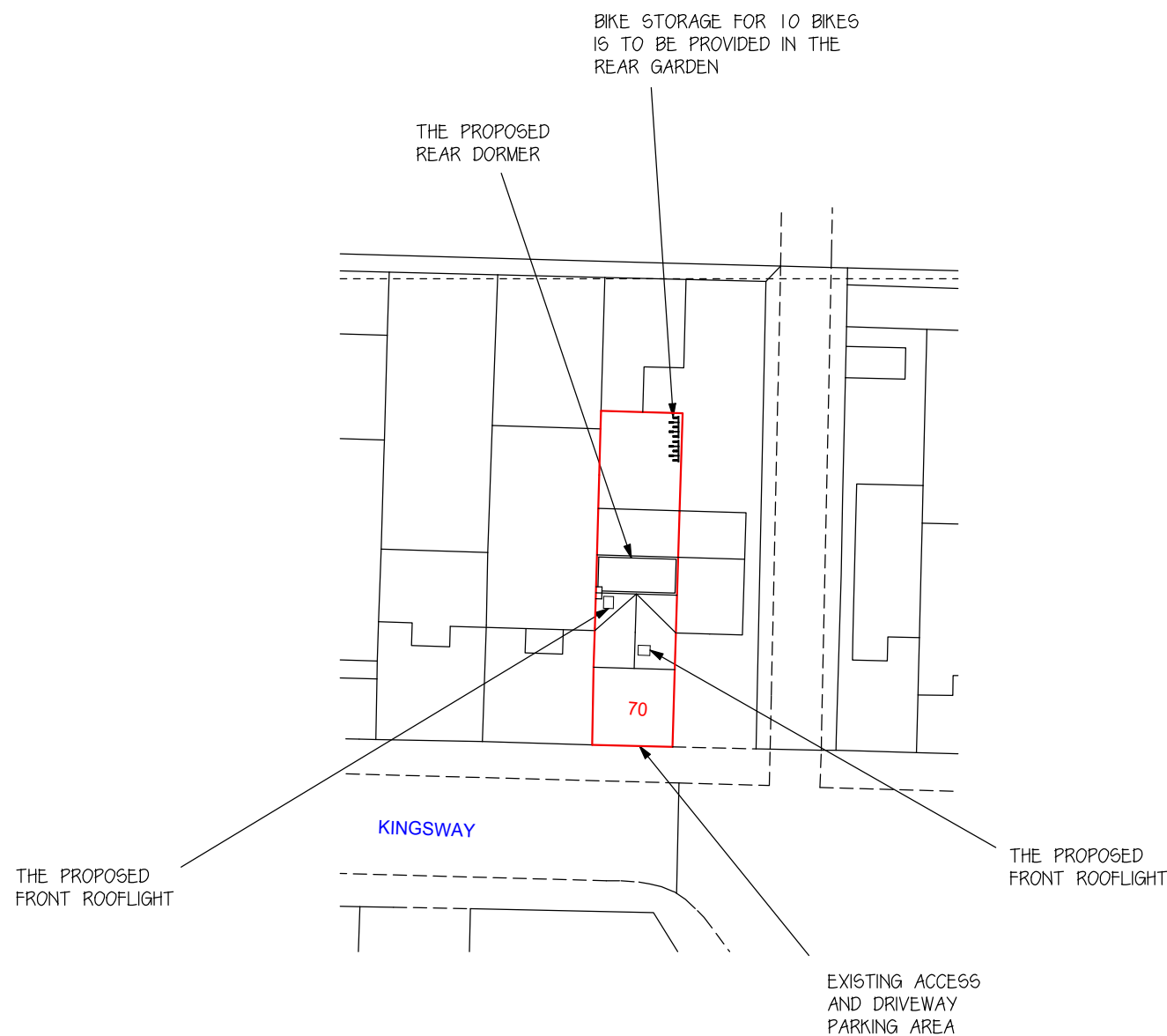
1:500 SITE PLAN
