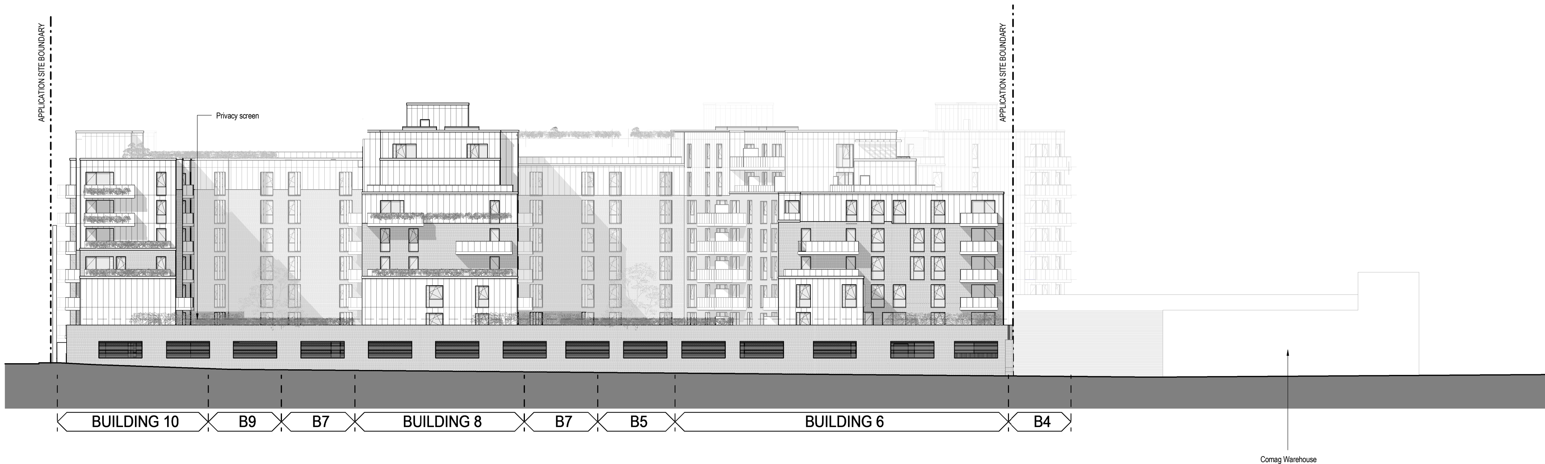
2 Elevation 06 1 : 250
