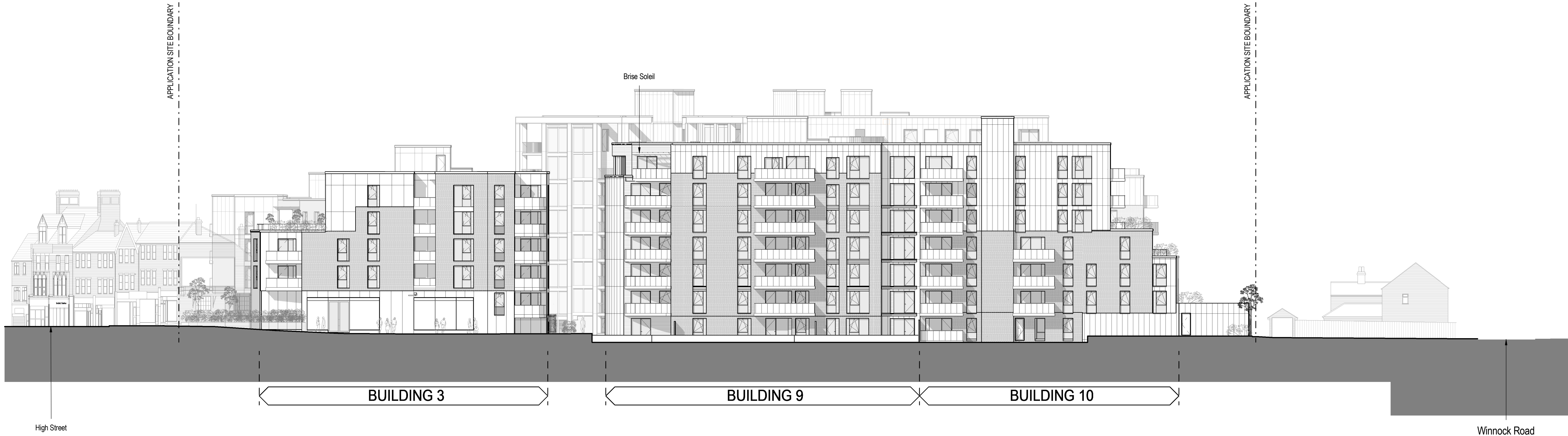
2 Elevation 03 1:250
