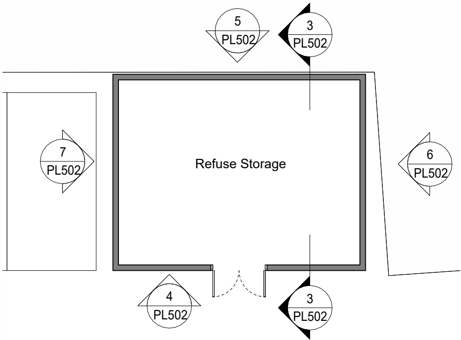
1 502- Refuse Storage 1 : 100
