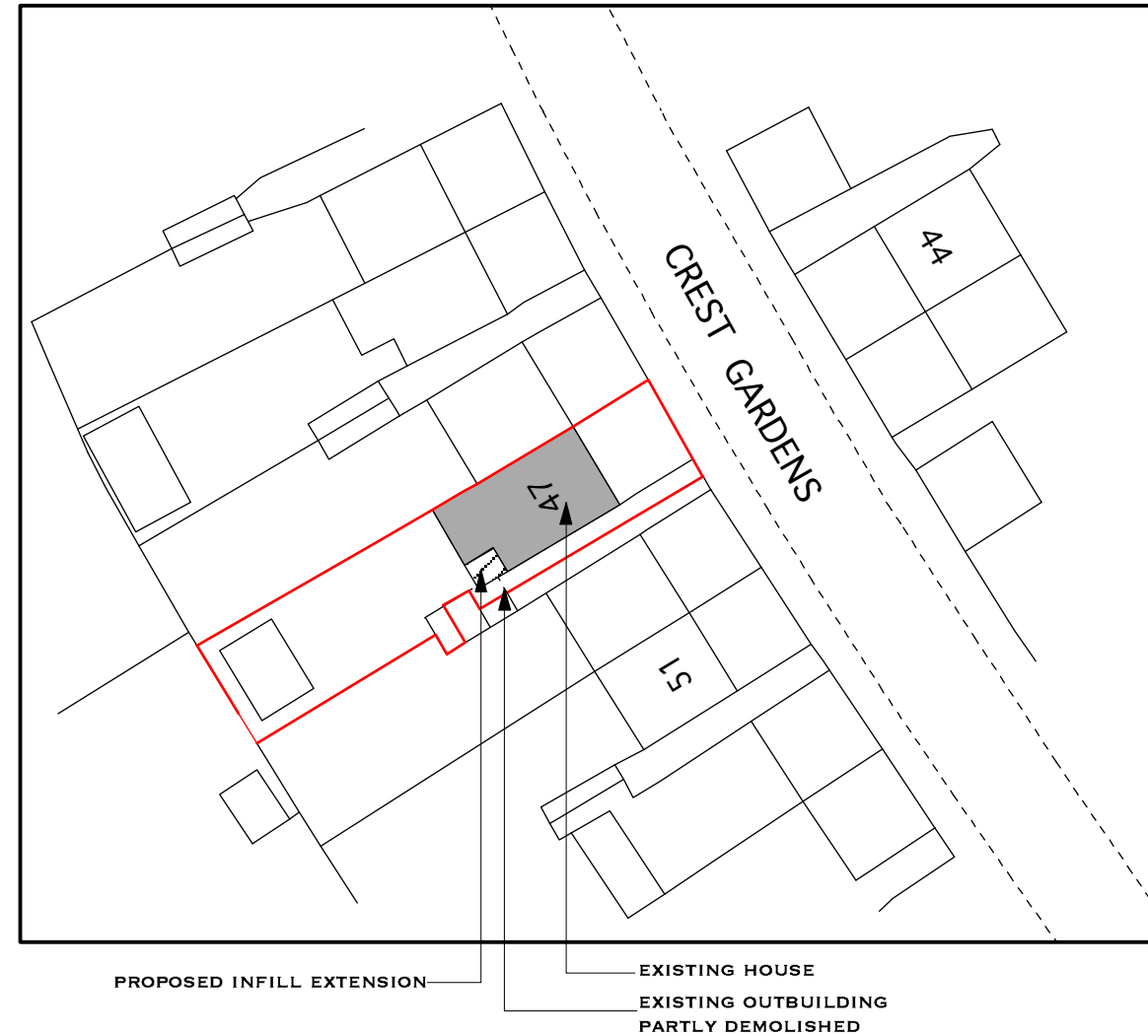
01 BLOCK PLAN A3 SCALE: 1:500
