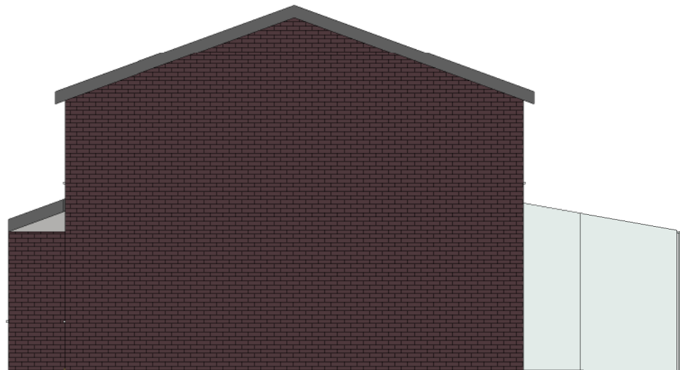
3 Side 1 1 : 100
