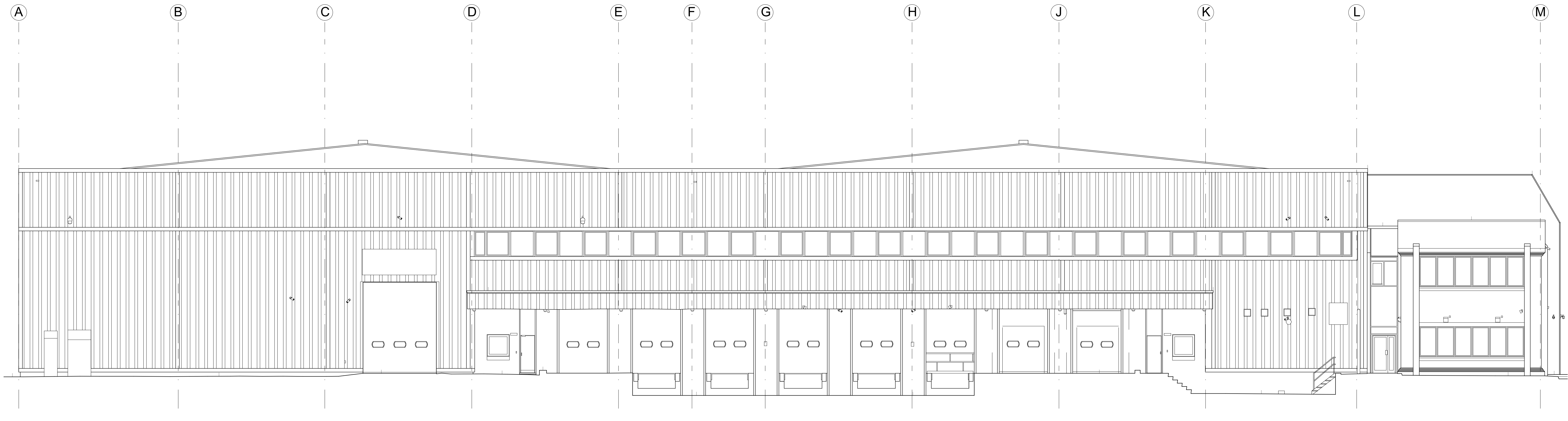
Elevation 01
