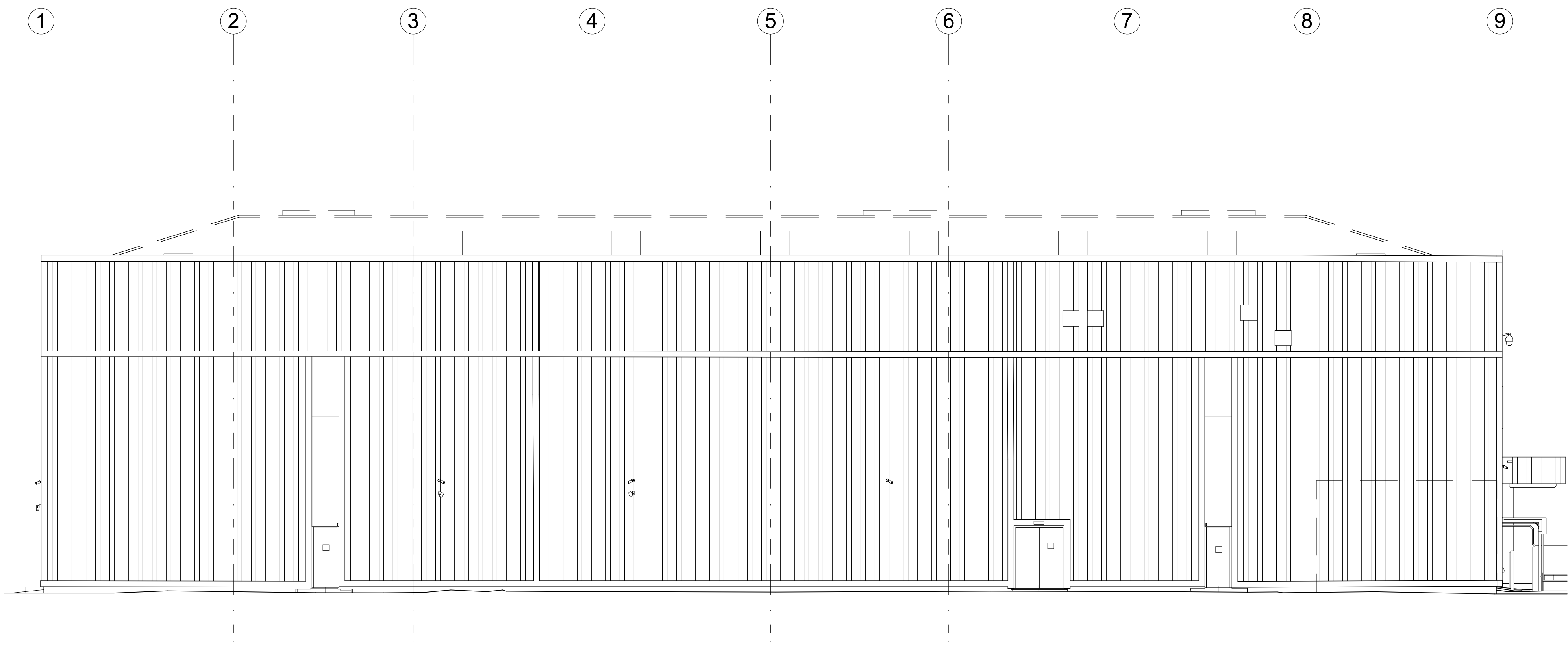
Elevation 02
