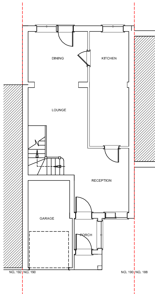
EIXISTING G/F (1:100)
