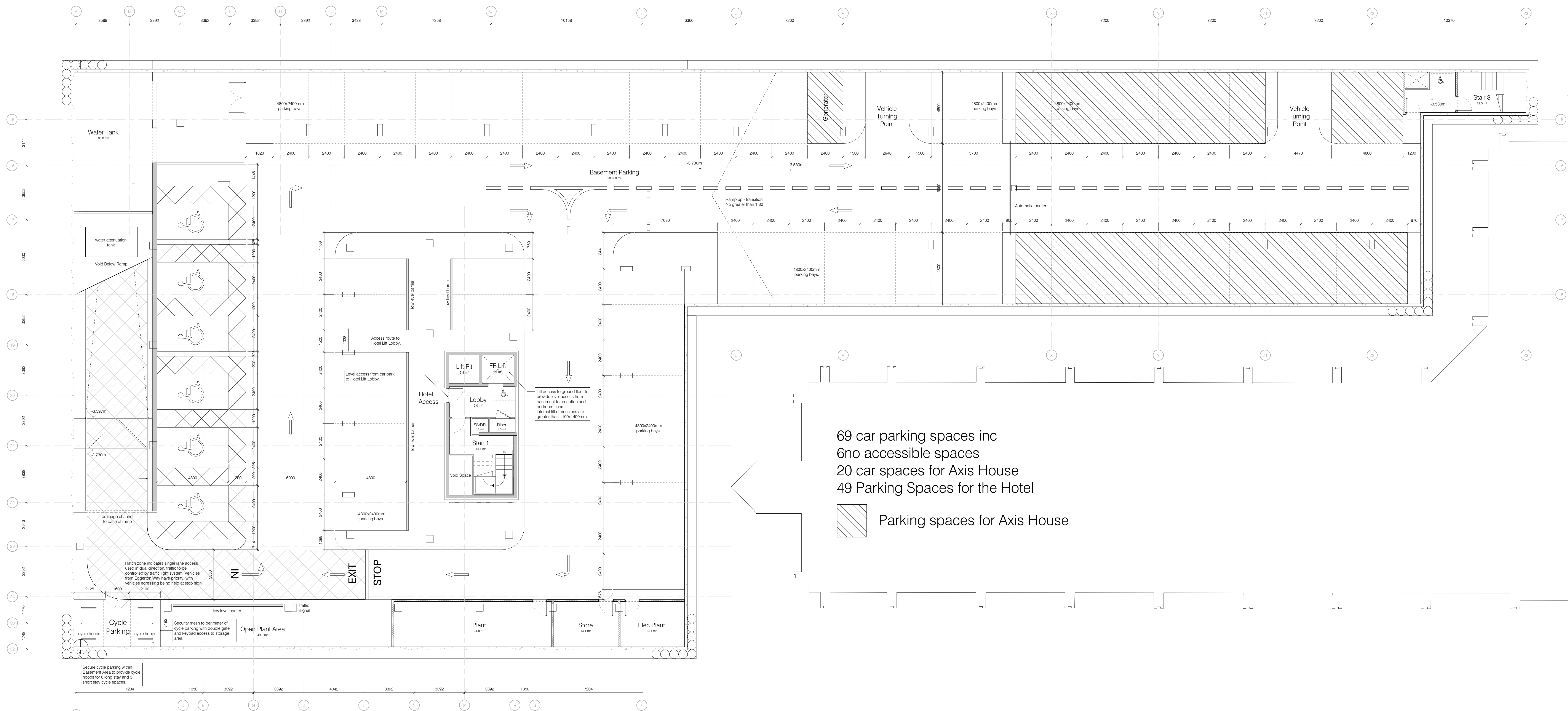
(90) Basement Scale: 1 : 100
