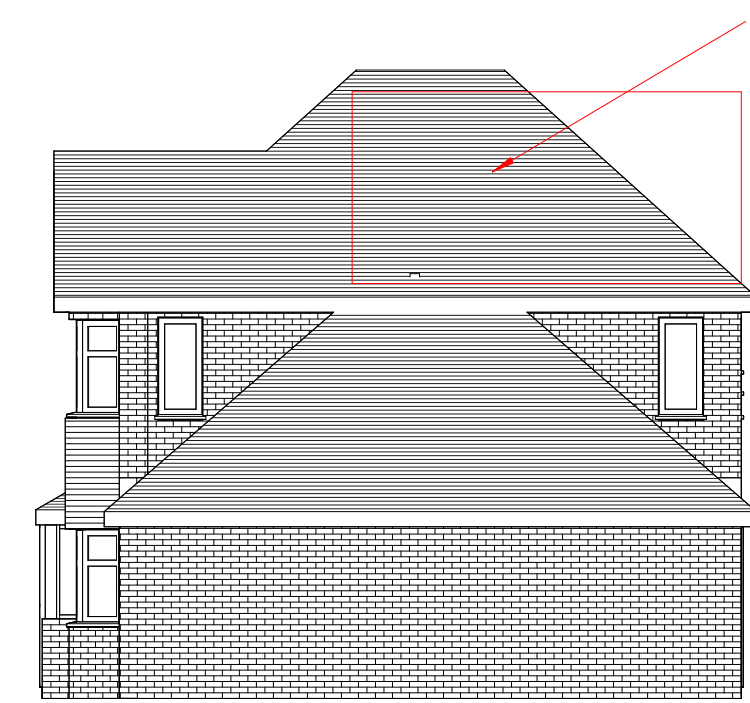
8 Right Elevation 1 : 100
