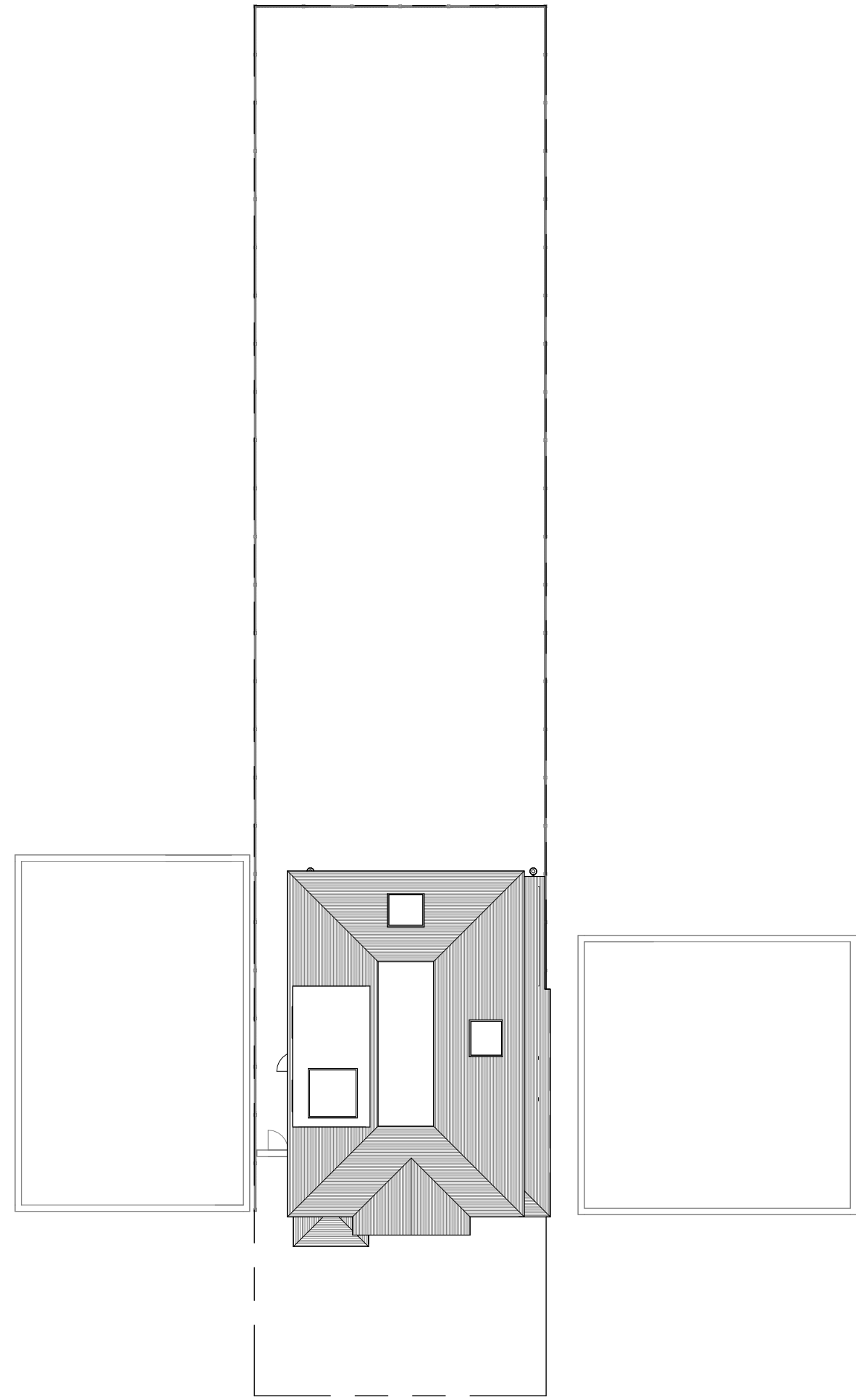
1 Site Plan 1 : 200
