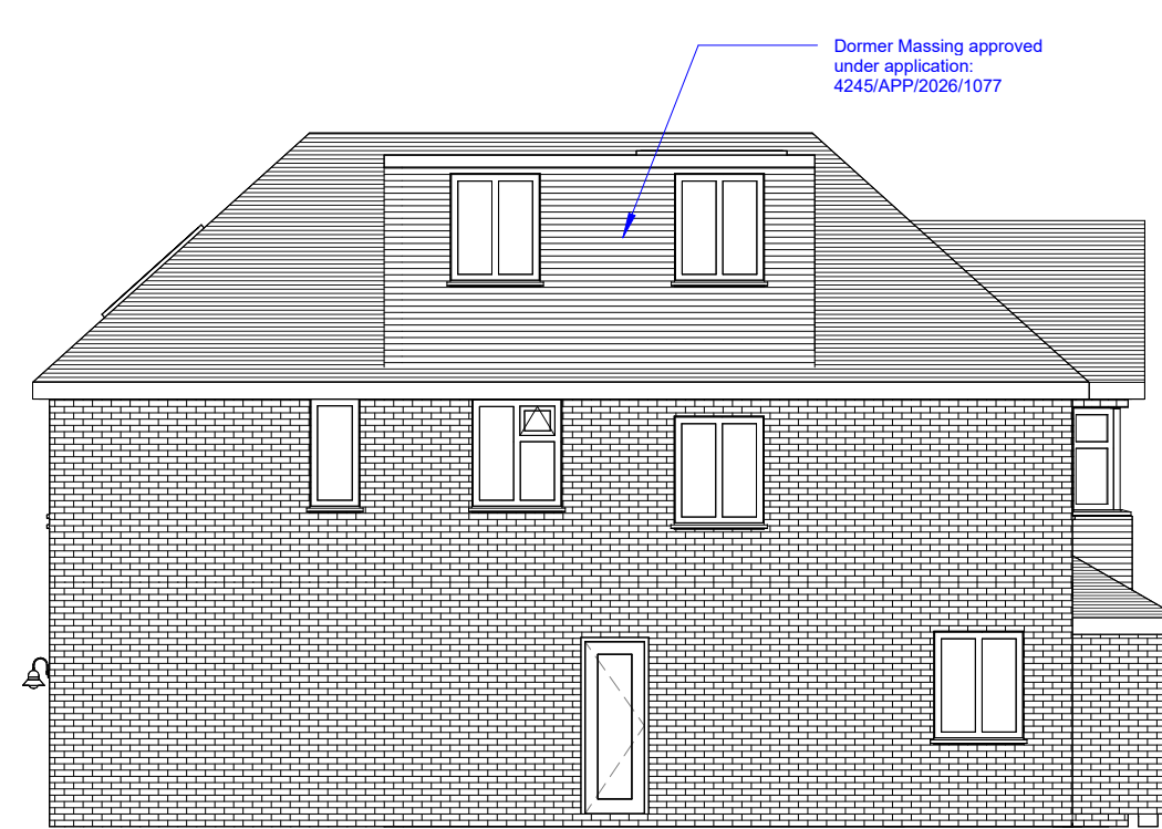
6 Left Elevation 1 : 100
