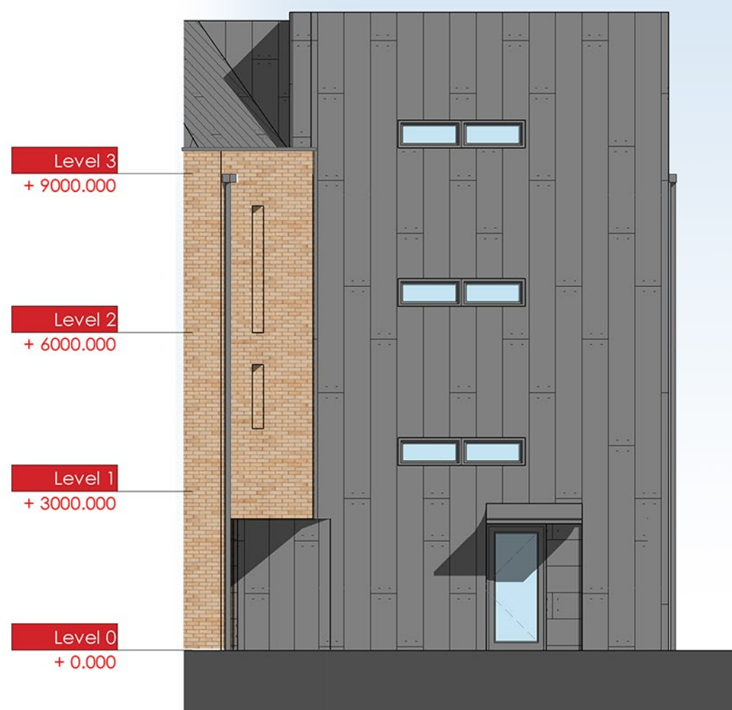
5 Elevation 5 1:100
