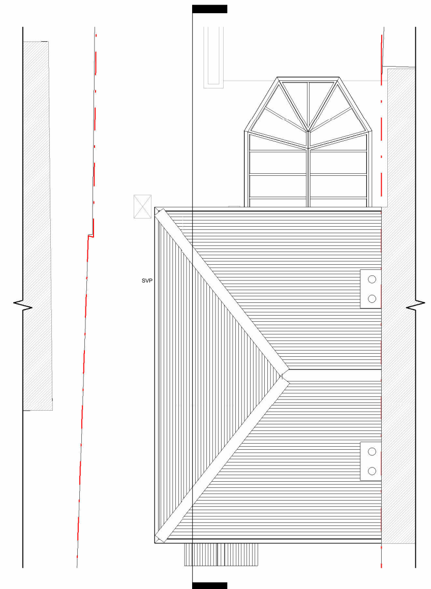
Roof Plan 1 : 100
