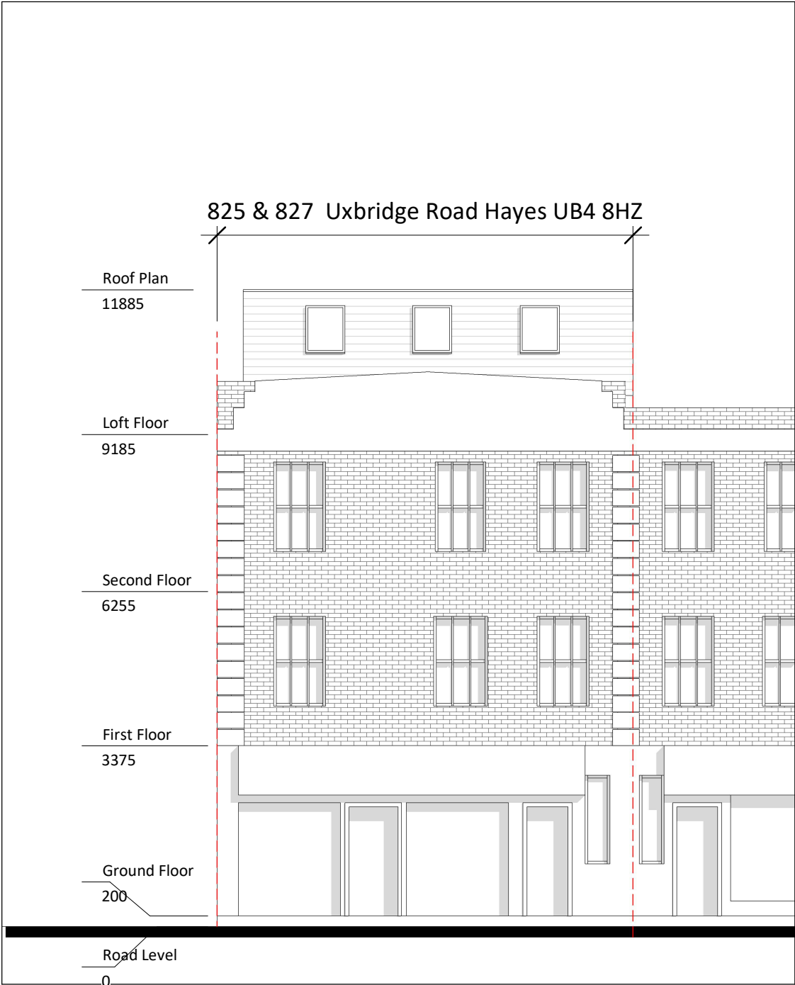
1 Front 1 : 100
