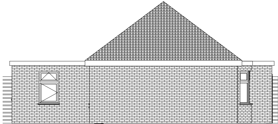
4 Left Elevation 1 : 100
