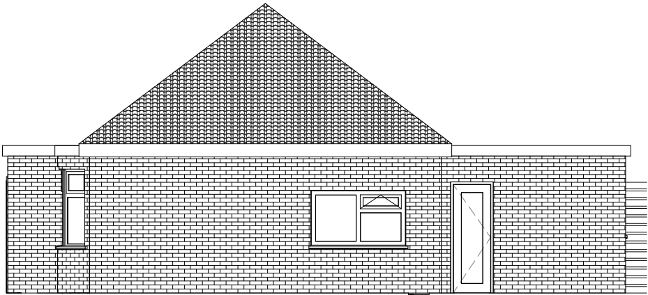
6 Right Elevation 1 : 100
