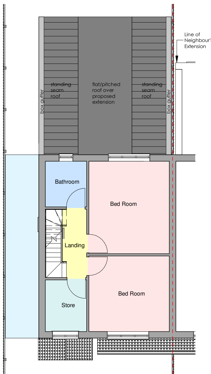
2 First Floor 2310-A-301 1 : 100
