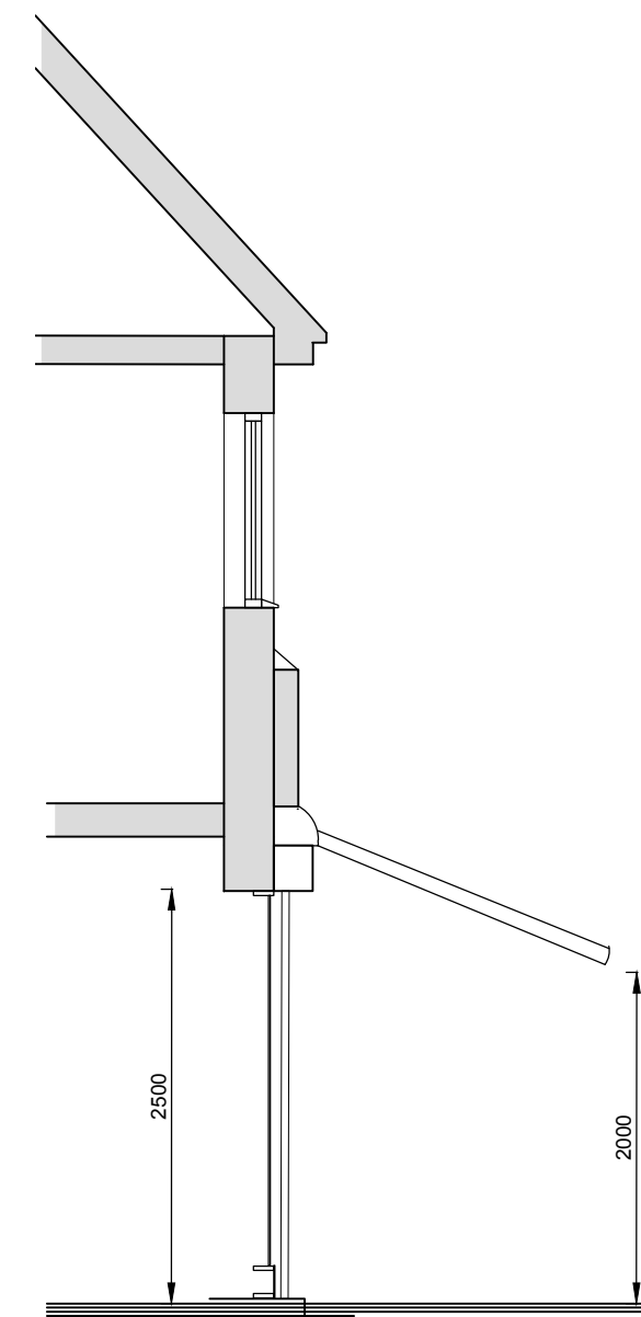
ELEVATION Scale: 1:50 @ A2
