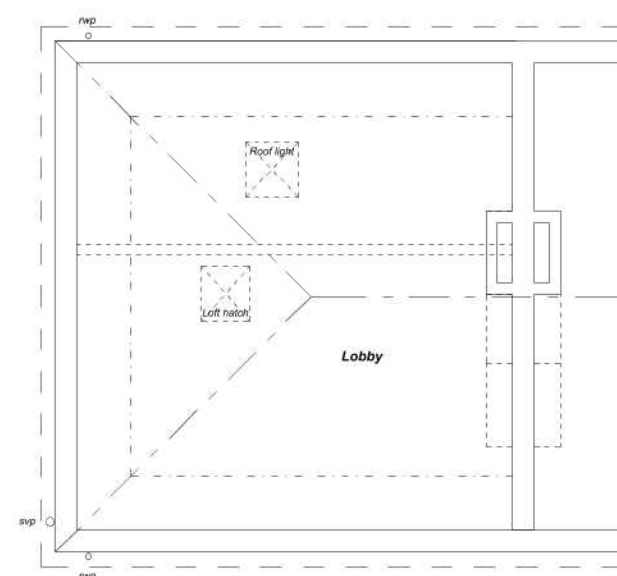
LOFT SPACE
