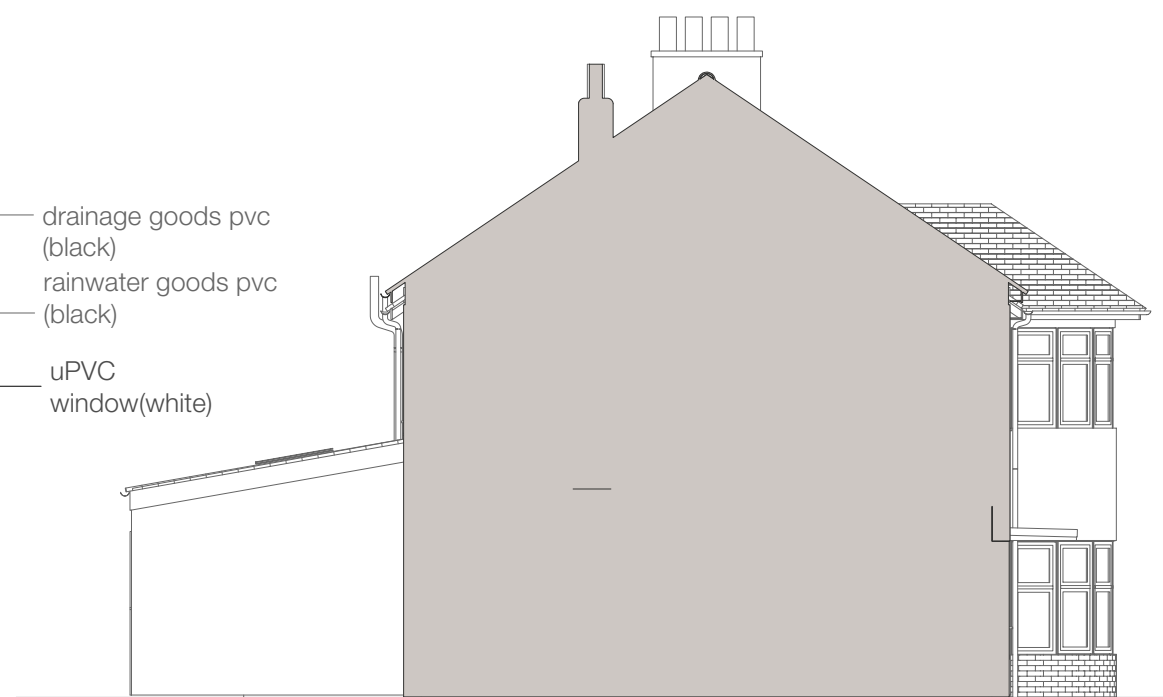
02 SIDE ELEVATION Scale: 1:100
