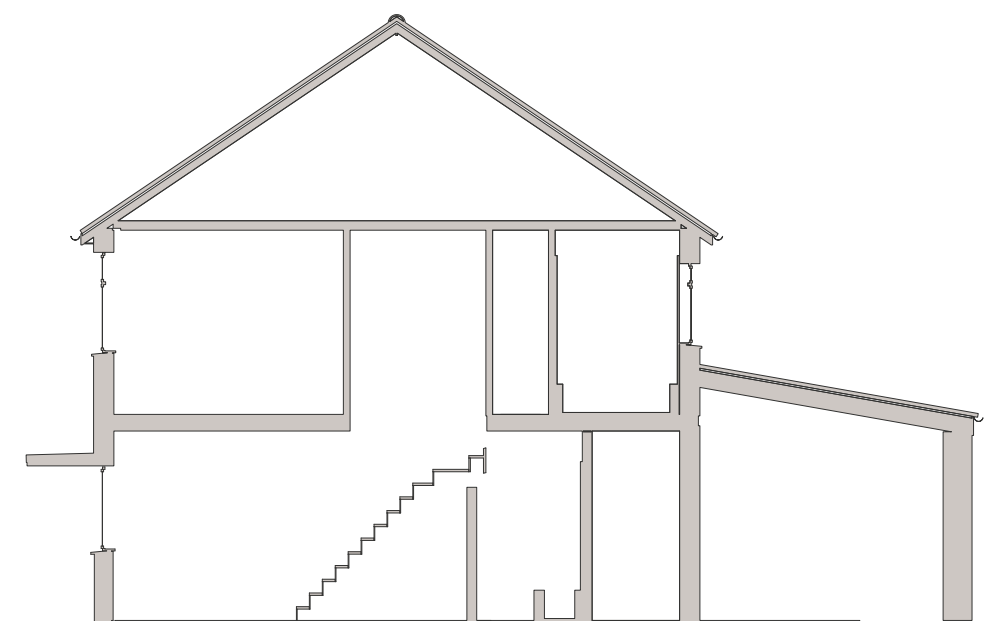
05 SECTION AA Scale: 1:100
