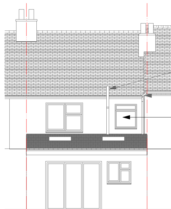
01 REAR ELEVATION Scale: 1:100
