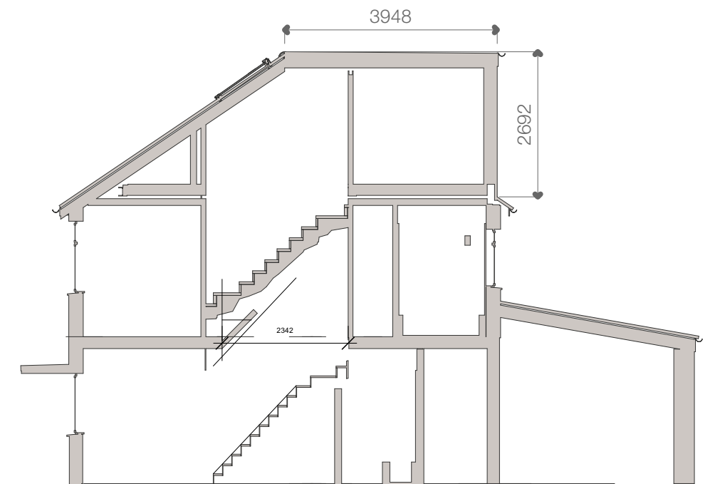
05 SECTION AA Scale: 1:100
