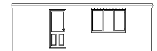
1:100 FLANK ELEVATION
