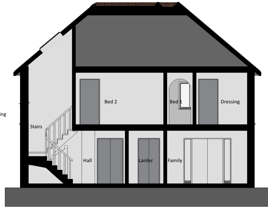
5 Section A-A
