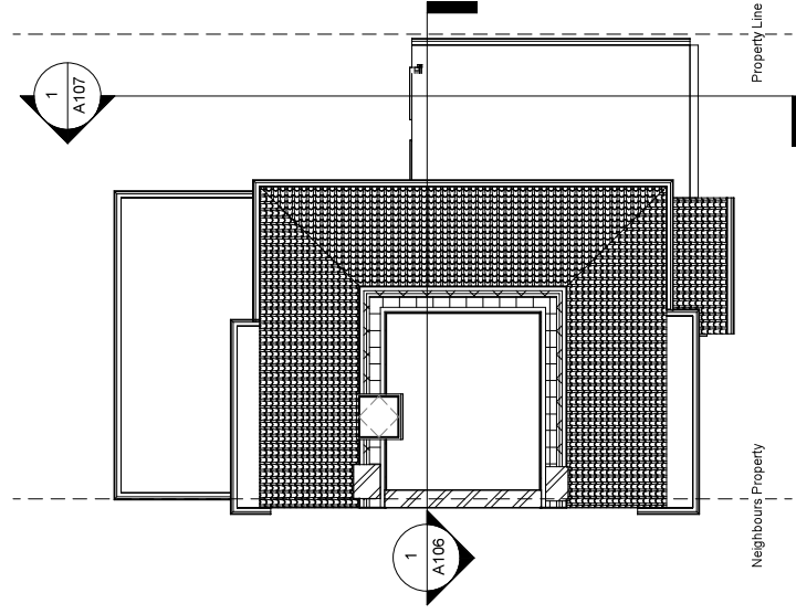
1 Loft - Existing 1 : 100
